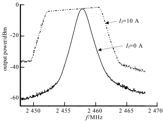
RBW=1 MHz,VBW=3 MHz, SPAN=20 MHz Fig.4 Spectrum of free oscillating magnetron 图4 自由振荡状态下磁控管输出频谱
